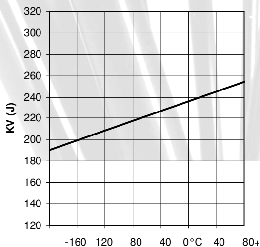
Curva di transizione solubilizz. a 1050°C Impact strength transition temperature
