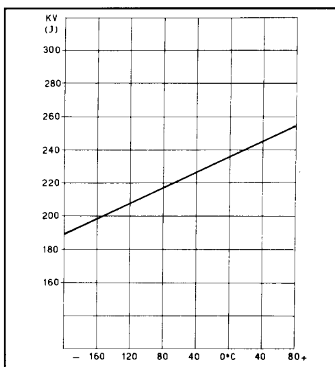
Curva di transizione Solubilizz. a 1050 °C Impact strength transition temperature
